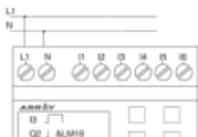
Fig 2.5 - Tipo AC
